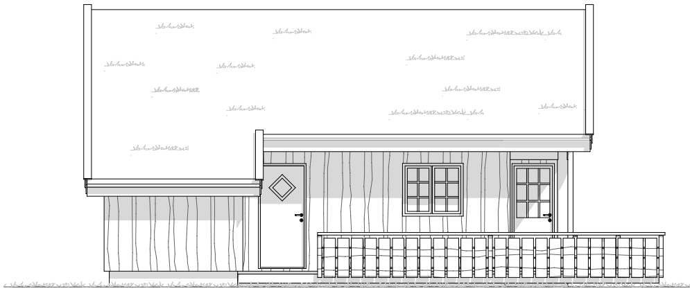
Fasade 1
