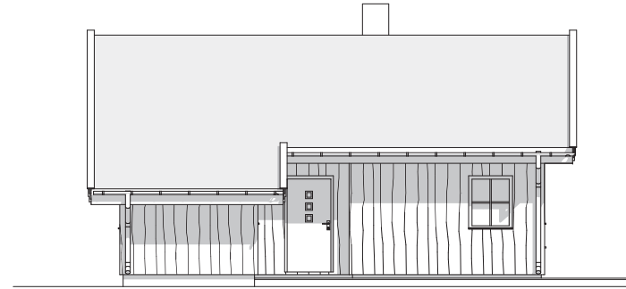
1:100 Fasade 1
