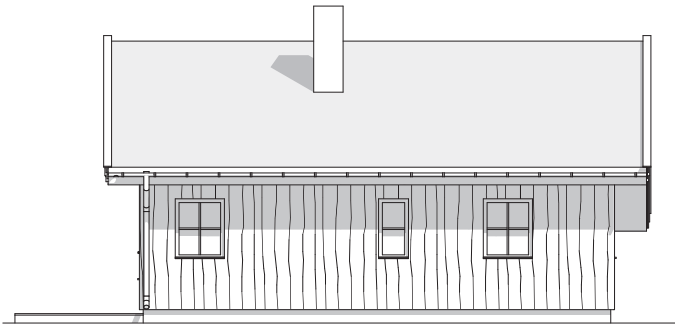
1:100 Fasade 3
