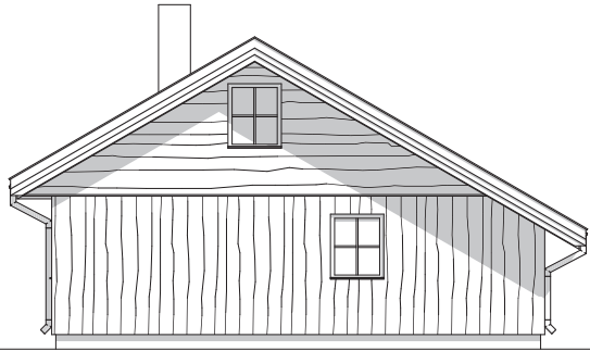
1:100 Fasade 2
