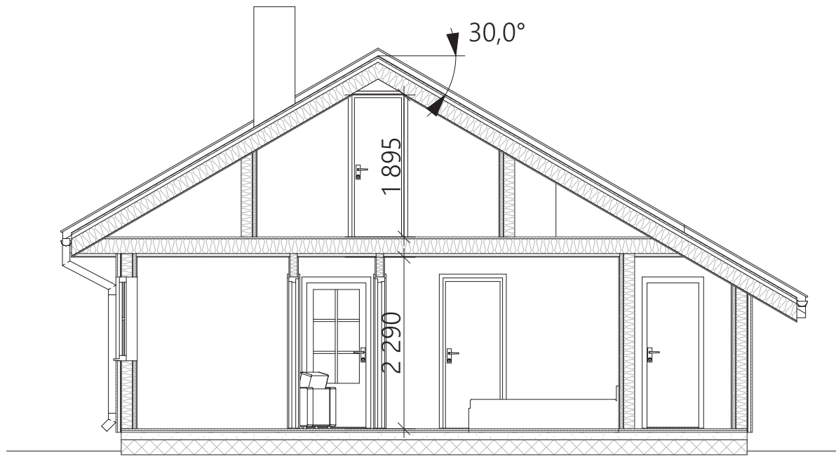
1:50 A
