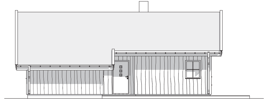
1:100 Fasade 1
